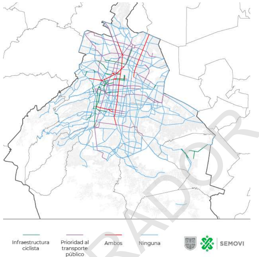
ILUSTRACIÓN 44. RED VIAL CON CARRILES DE CIRCULACIÓN CICLISTA O DE VEHÍCULOS DE TRANSPORTE PÚBLICO
